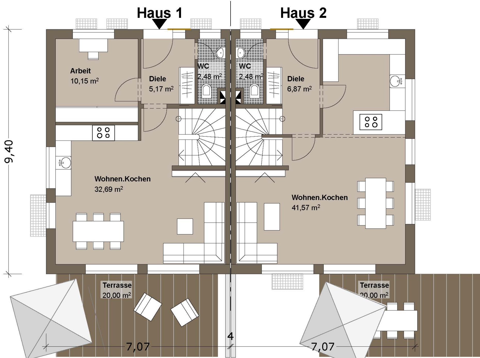
Robert-Koch-Straße Grundriss Erdgeschoss alternativ
