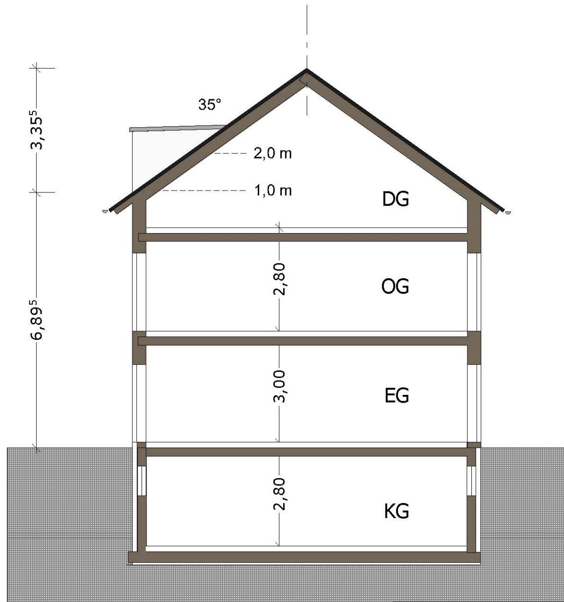
Robert-Koch-Straße Schnitt
